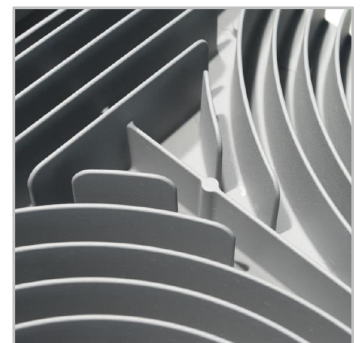
Om een optimaal thermisch beheer in warme omstandigheden te garanderen is de AVENTO uitgerust met grote koelvinnen
